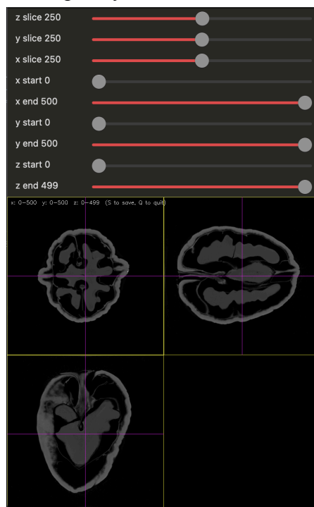
Рис. 4, Программа bounds_gui.py
